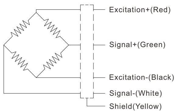
Wiring Code@Clockwise
